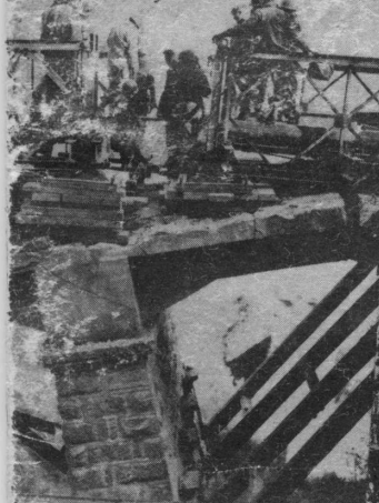
Leaning-pier Bailey - Castel di Castro
